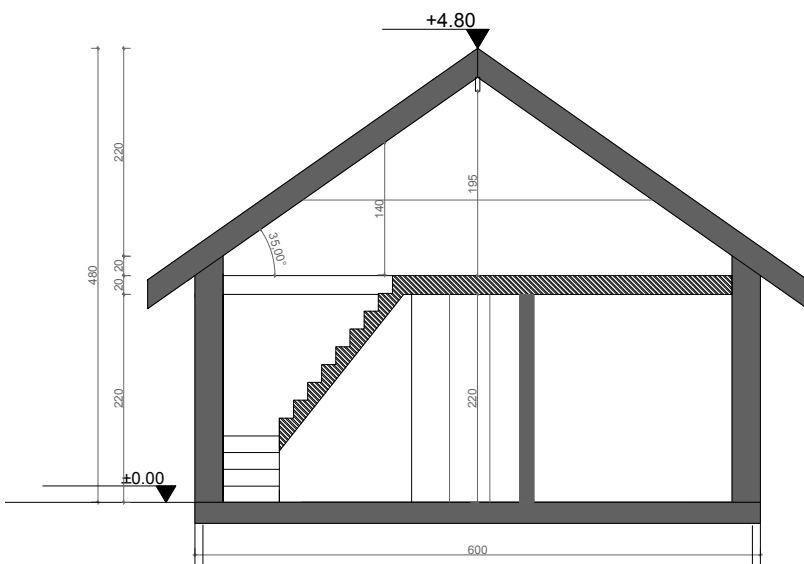
PRZEKRÓJ A-A
